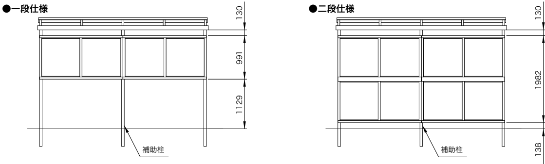
パネル枠幅＝テラスたる木外々
