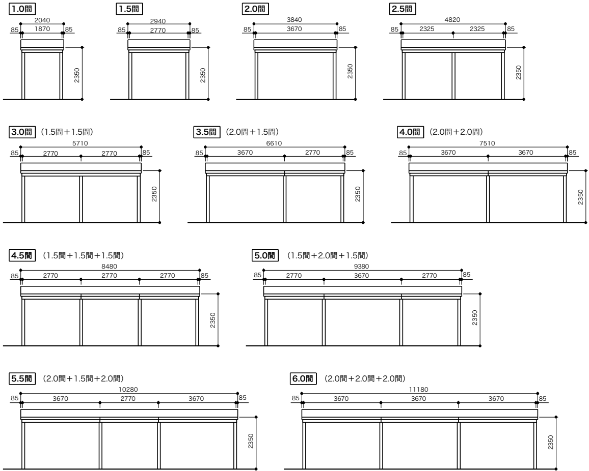
■間口別 概略寸法図
