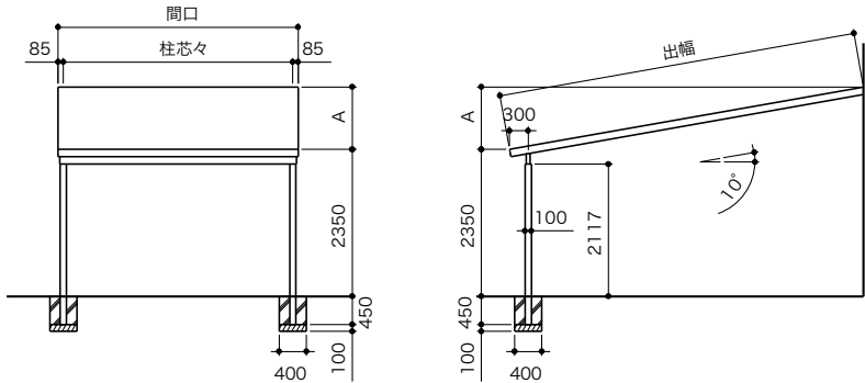
■ A 寸法表 (mm)
