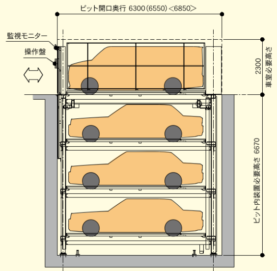
側面図
