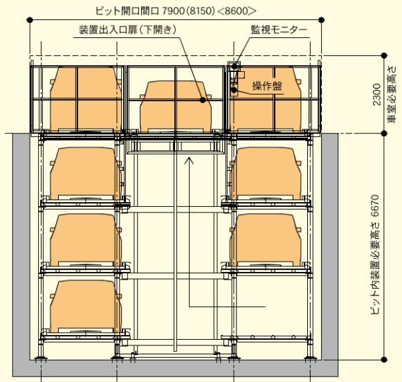
正面図
