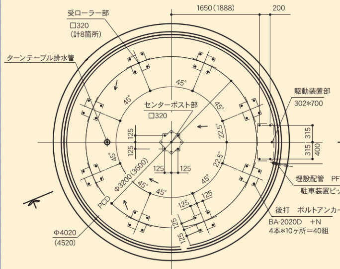
ターンテーブル ピット平面図
