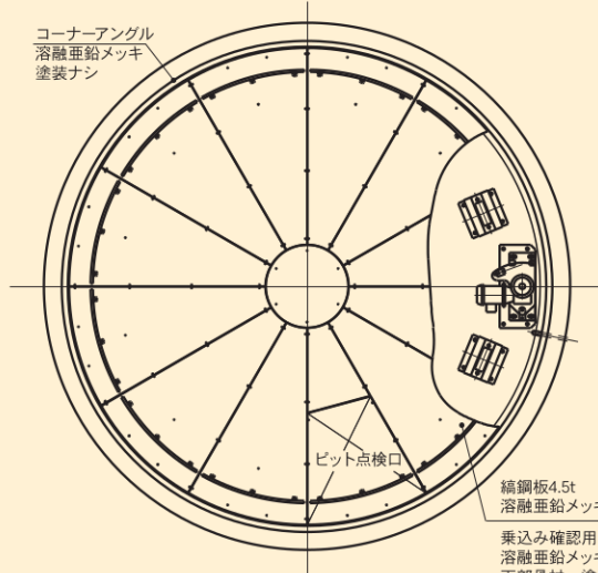
ターンテーブル 平面図
