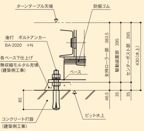
ベース部(受ローラー) 詳細図
